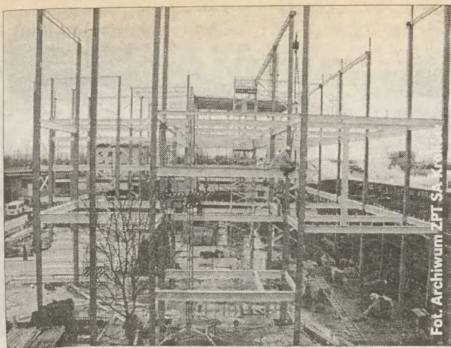
Powstaje hala, w której będzie jedyna w Europie Środkowej linia do produkcji tytoniowej krajanki ekspandowanej
