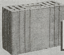
CEGLA MODULARNA Z UCHWYTEM kl. 150 zastosowanie: - ścianki działowe - ściany warstwowe, zewnętrzne - ściany osłonowe - ściany wypełniające
