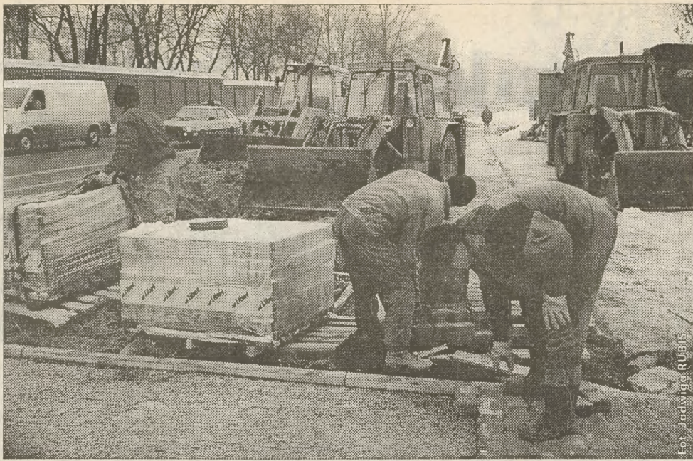
Na skrzyżowaniu ul. Lublańskiej i 29 Listopada trwają „kosmetyczne” prace przy układaniu kostki brukowej. Budowlańcy są gotowi pracować nawet przy temperaturze -15 stopni Celsjusza. (JR)
