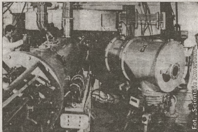
Ośrodek badawczy w Dubnej koło Moskwy — fragment aparatury służącej do „produkcji” nowych pierwiastków chemicznych
