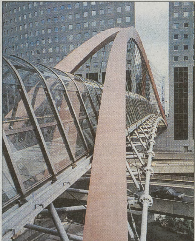
Kryta stalowa kładka dla pieszych w dzielnicy La Défense w Paryżu.
