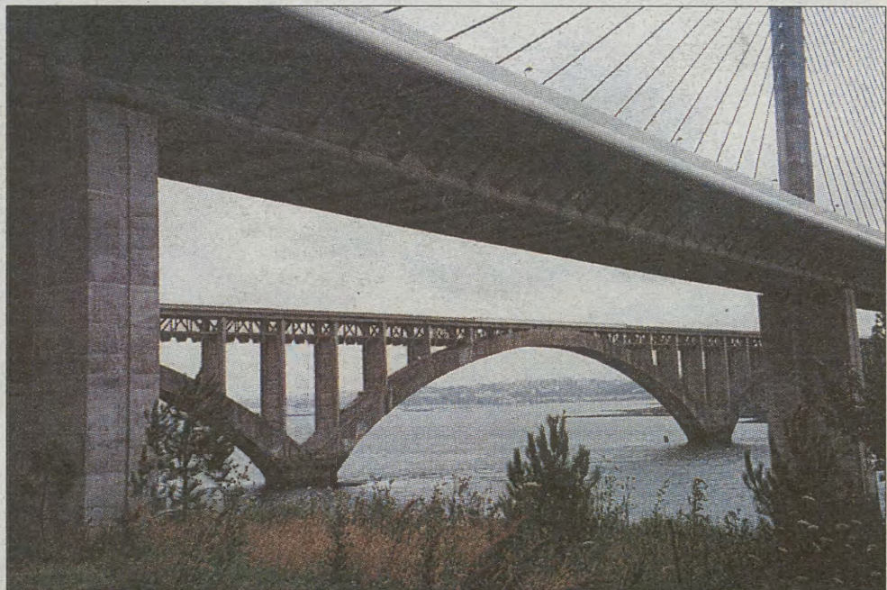
Dwa mosty na rzece Elorn w Bretanii; stary żelbetonowy łukowy 3-przęsłowy o rozpiętości przęsła 186,4 m i nowy podwieszony, 2-pylonowy o rozpiętości głównego przęsła 400 m.
