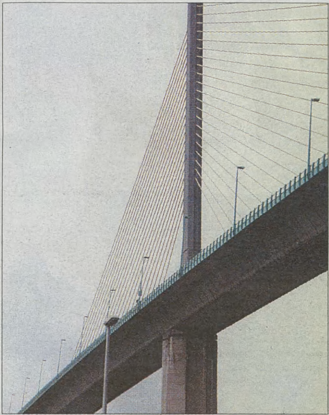
Pylony i zakotwienia cięgien podwieszających w moście Normandii, u ujścia Sekwany
