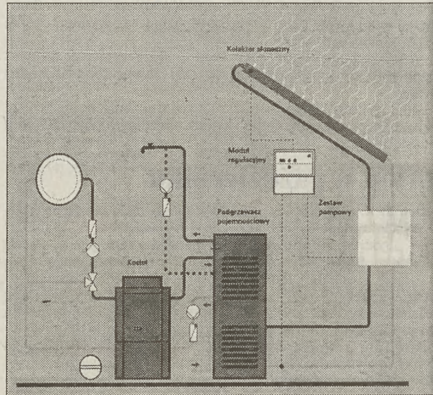
Schemat dwurzędowego podgrzewania z kolektorem słonecznym, podgrzewaczem dwuobiegowym i zestawem pompowym
