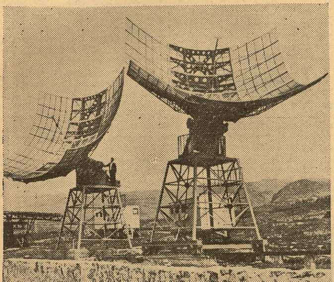
Wielki radioteleskop w Byurakańskim Obserwatorium Astronomicznym (Armeńska SRR) służy do badania promieniowania obiektów kosmicznych w granicach naszego systemu słonecznego oraz radio-promieniowania słońca i mgławic pozagalaktycznych.
