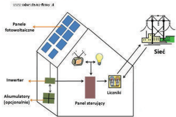
Instalacja fotowoltaiczna- schemat. Źródło Internet.
