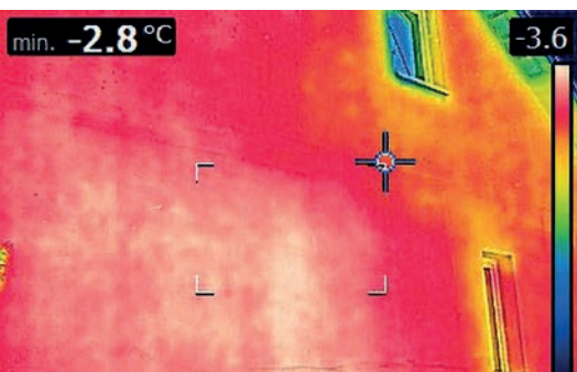
Źle zaizolowana przegroda pionowa
