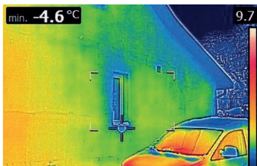
Dobrze zaizolowana przegroda pionowa
