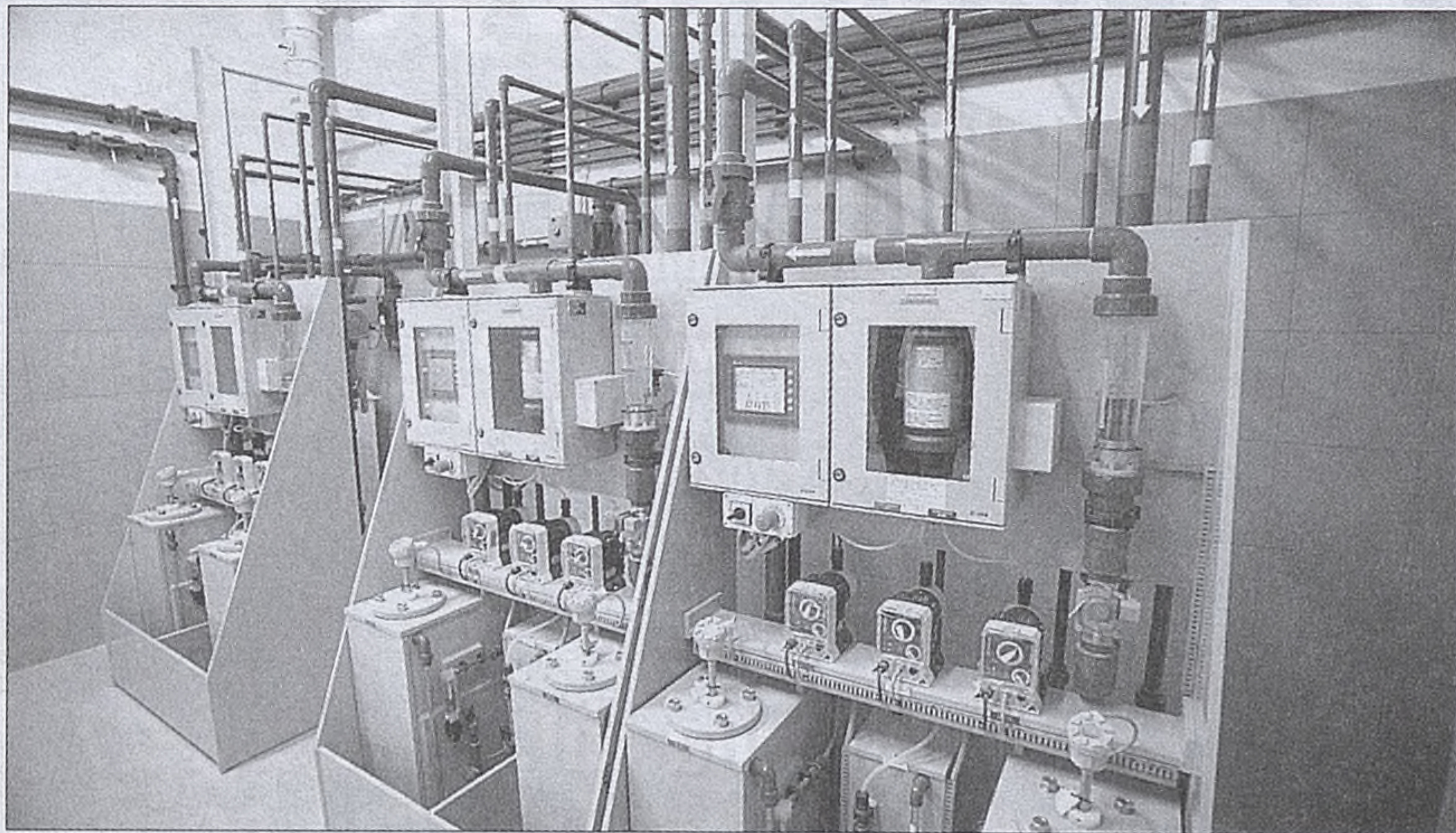
Generatory dwutlenku chloru w Budynku Chemii i Dezynfekcji
