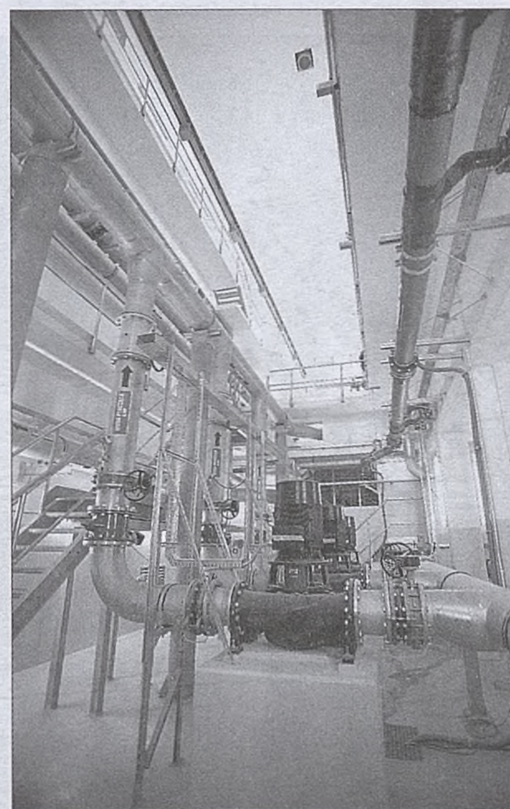
Pompownia wody płucznej
