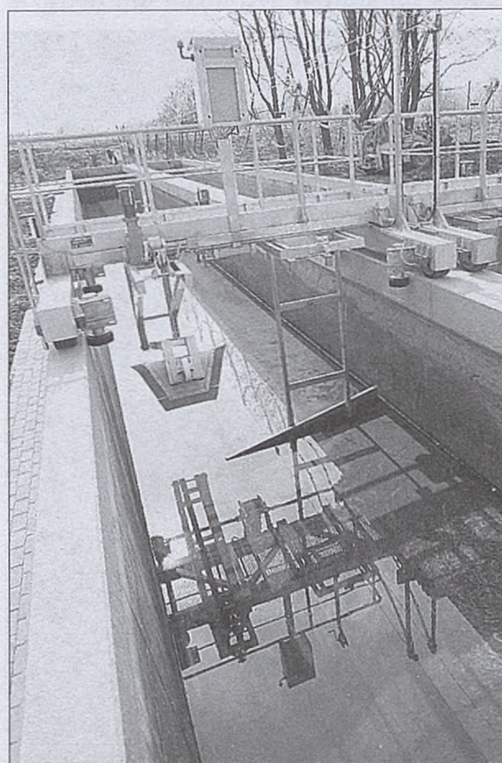
Odmulnik – automatyczny zgarniacz osadów
