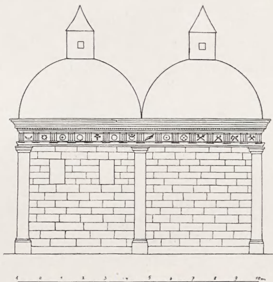
Fig. 74. Kalwaria Zebrzydowska. Pierwotny kościół Ukrzyżowania. Zrekonstruował J. Szablowski.
