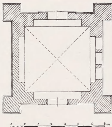
Fig. 78. Kalwaria Zebrzydowska. Brama wschodnia. Rzut poziomy. Zdjmował J. Szablowski.
