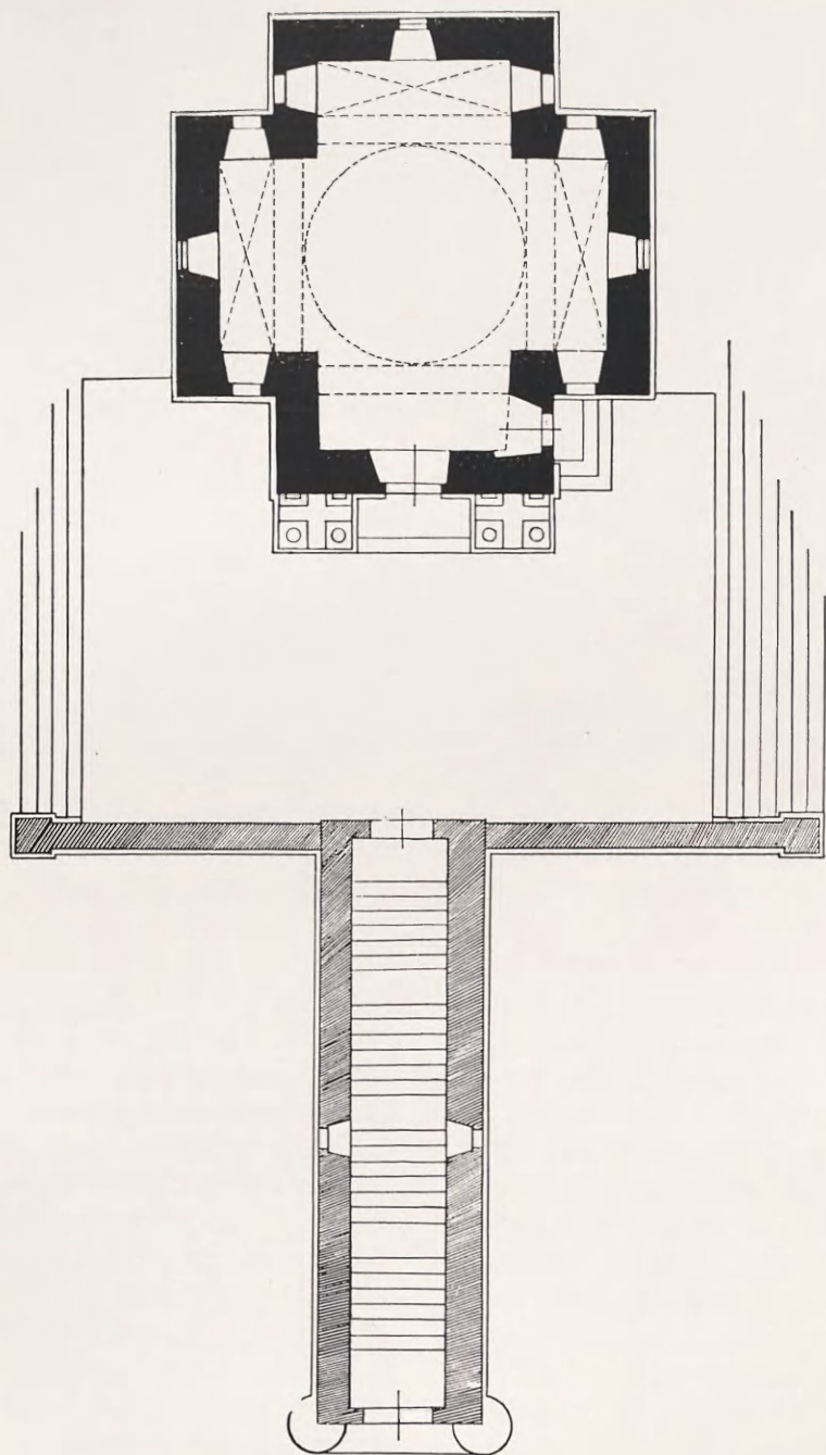
Fig. 21. Kalwaria Zebrzydowska. Ratusz Piłata i Święte Schody. Rzut poziomy. Zdejmował J. Szablowski.
