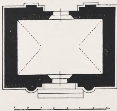
Fig. 54. Kalwaria Zebrzydowska. Brama Zachodnia. Rzut poziomy. Zdejmował J. Szablowski.
