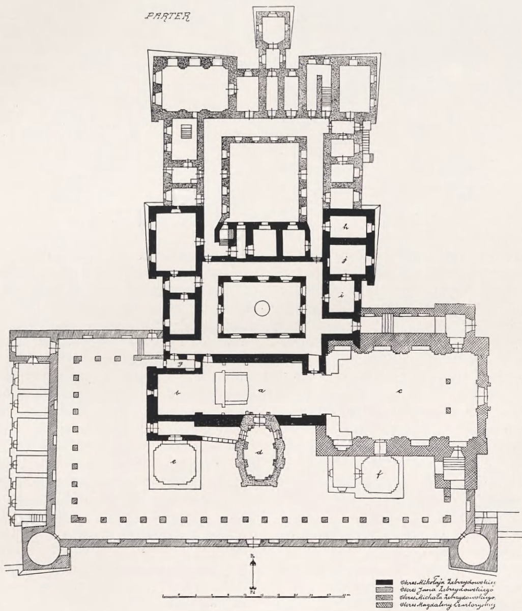
Fig. 4. Kalwaria Zebrzydowska. Kościół i klasztor oo. bernardynów. Rzut poziomy parteru.
