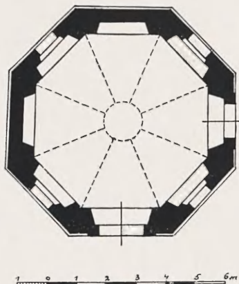
Fig. 47. Kalwaria Zebrzydowska. Wniebowstąpienie. Rzut poziomy. Zdejmował J. Szablowski.
