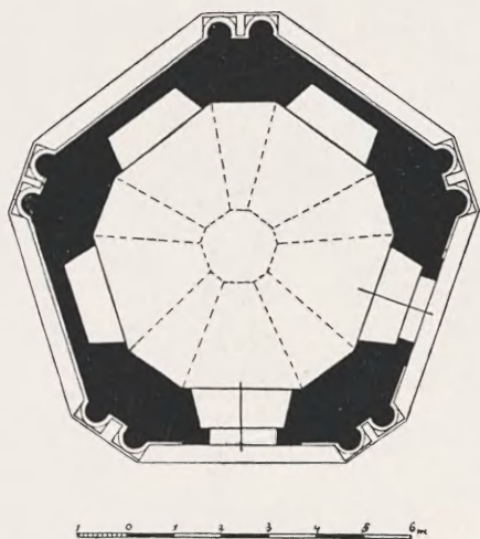
Fig. 29. Kalwaria Zebrzydowska, Ogrojec. Rzut poziomy. Zdjęmował J. Szablowski.
