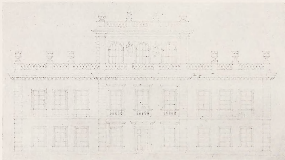
Fig. 12. Obserwatorium Astronomiczne, fasada od ul. Kopernika. Rysunek inż. Rossmanna z r. 1814 w Zbiorze Graficznym Biblioteki Jagiellońskiej.
