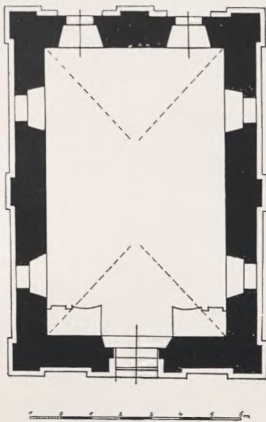
Fig. 49. Kalwarja Zebrzydowska. Wieczernik. Rzut poziomy. Zdejmował J. Szablowski.
