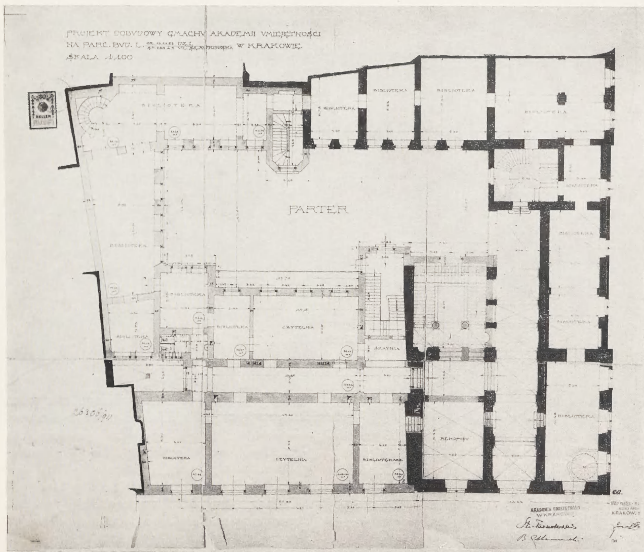
9. Rozbudowa gmachu Akademii Umiejętności wg projektu J. Pakiesa i W. Krzyżanowskiego, parter, ok. 1911
