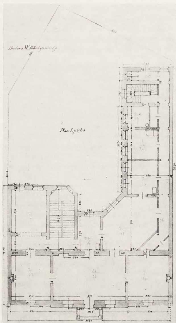
11. Dom Pokutyńskiego przy ul. Karmelickiej 29, plan pierwszego piętra
