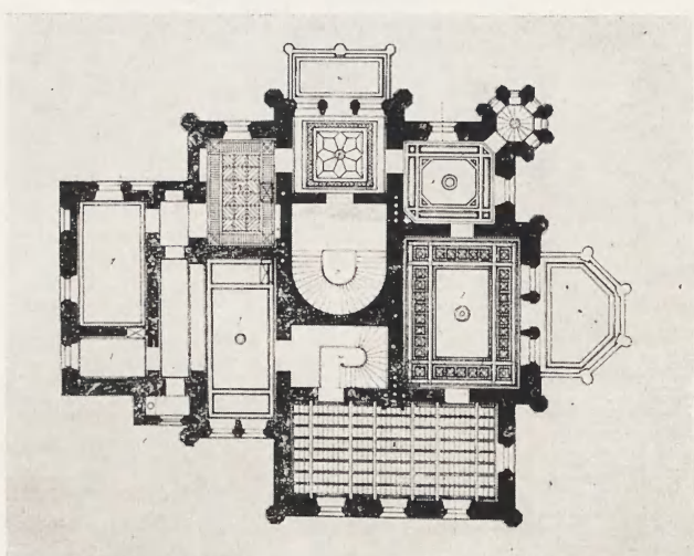
2. Parter i pierwsze piętro willi w Piekarach
