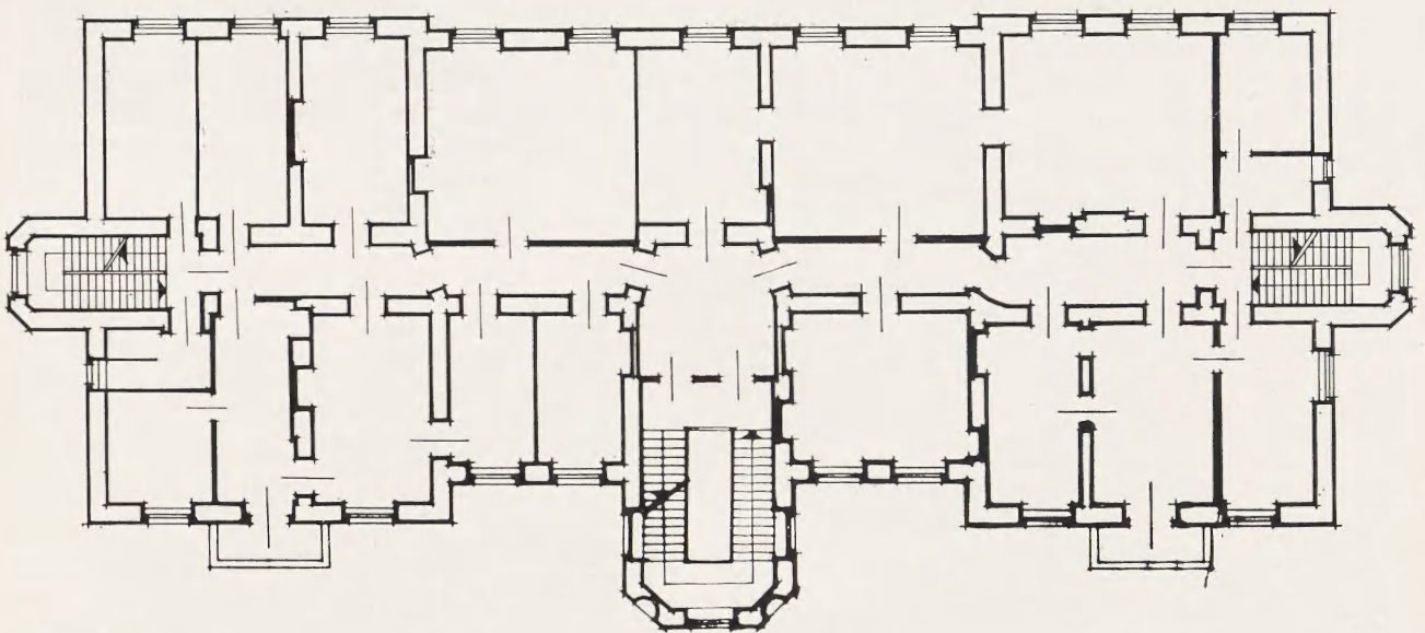
3. Pałac Puszetów, rzut pierwszego piętra. Rys. P. Stępień
