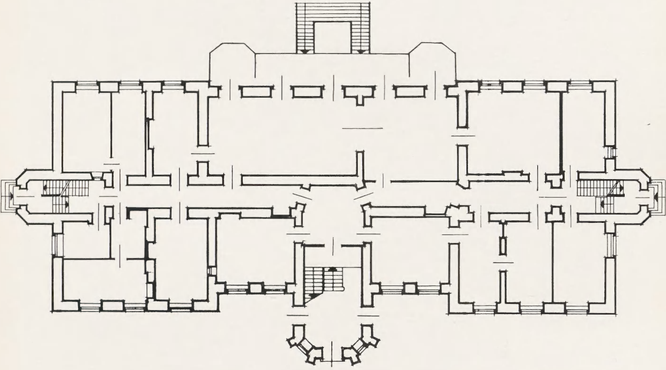
2. Pałac Puszetów, rzut parteru. Rys. P. Stępień
