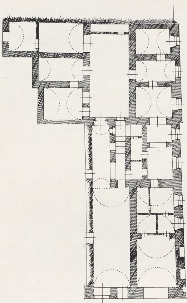
Plan parteru — stan obecny
