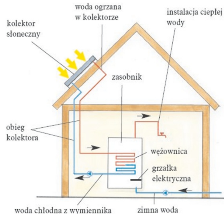
Schemat działania kolektora słonecznego
