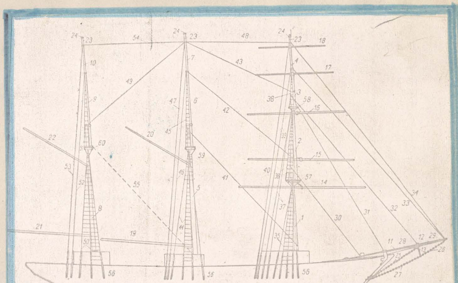
Omasztowanie i olinowanie stałe (barkentyna)
