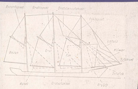
Ożaglowanie gafflowe
