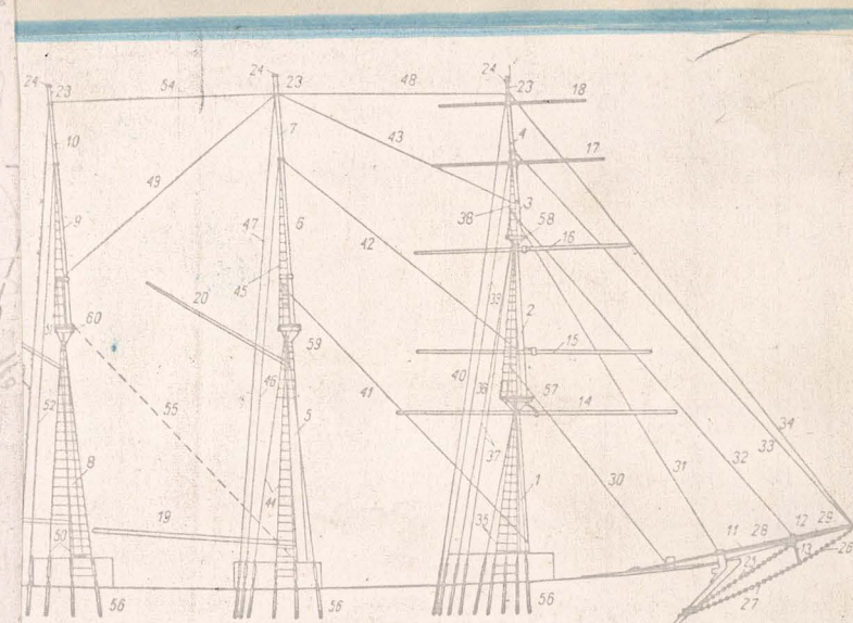
Omasztowanie i olinowanie statku (barkentyna)
