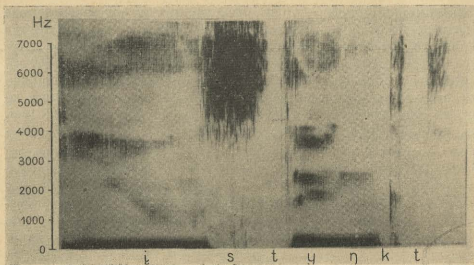
Ryc. nr 6: Spektrogram wyrazu istynkt .
