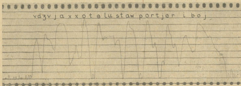
Fig. 4. Overall level curve of the sentence W drzwiach hotelu stał portier i boi.
