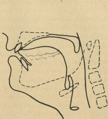
Ryc. nr 1: Rentgenogram statyczny przedłużanej głoski t .
