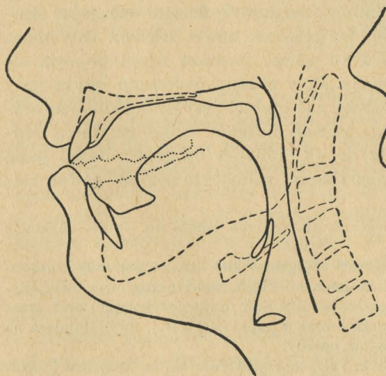
Ryc. nr 2: Rentgenogram statyczny przedłużanej głoski v .
