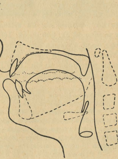
Ryc. nr 4: Fragment (1 klatka) kino-rentgenogramu głoski v z wyrazu vøš (zwierzę).
