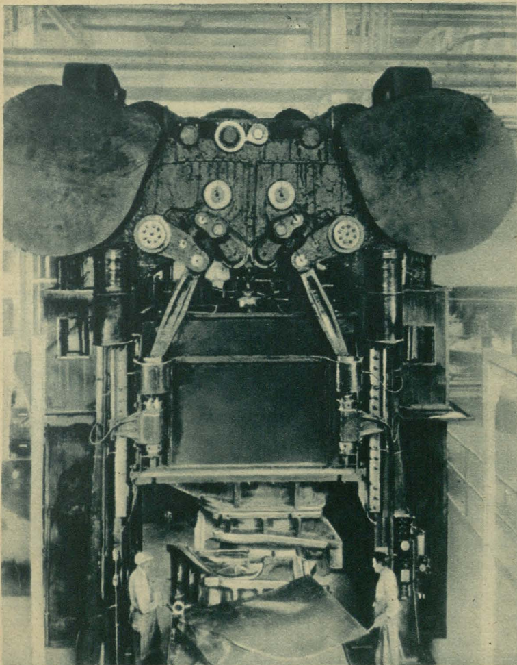
PRASA OLBRZYM. Oto jedna z potężnych pras w zakładach Forda w Detroit służących do wytłaczania z blachy stalowej całych części karoserji.
