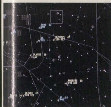
Widok na radarze wtórnym. Widać „echa” samolotów i chmury (kropki po lewej)
