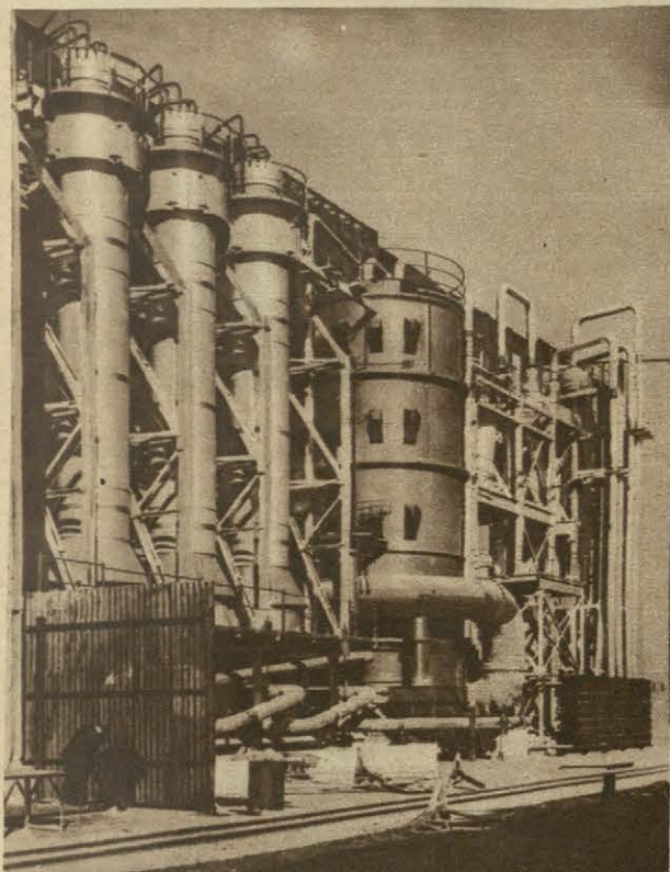
NAFTA Z WĘGLA. W wielkich zakładach przemysłowych Imperial Chemical Industries w Billingham w Anglii przetwarza się obecnie węgiel w cenniejszą jeszcze w dzisiejszych czasach naftę. Imponujący jest widok olbrzymich aparatów do tego celu.
