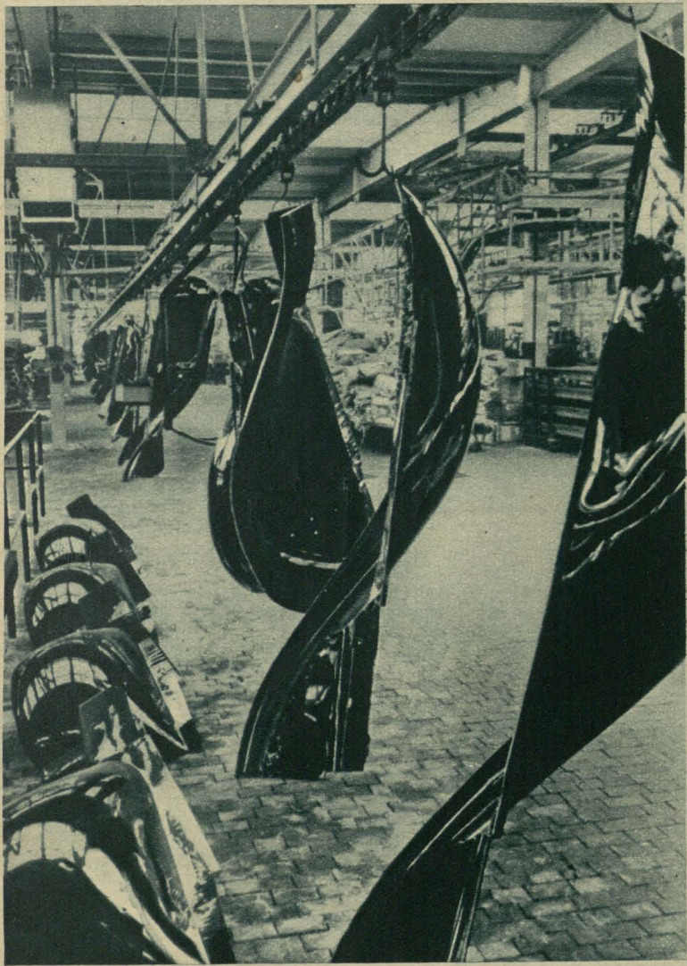
TASMOWA PRODUKCJA BŁOTNIKÓW AUTOMOBILOWYCH. Pięć kilometrów długości ma taśma, która w wielkiej fabryce samochodowej pod Berlinem wyrzuca zupełnie gotowe błotniki, dające się bezpośrednio potem założyć do wozów.
