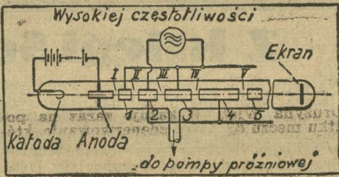
Oto schemat urządzenia Wideroe'a do „wywindywania” promieni katodowych na większą szybkość.
