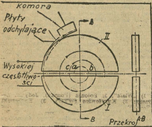
Schemat aparatury Lawrence i Livingstone'a do wywoływania pedu cząsteczek odpowiadającego napięciu milionów volt.
