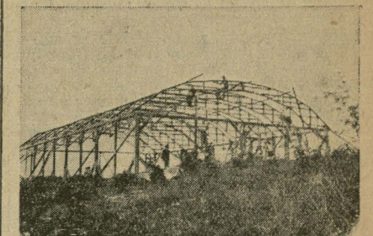
W Tegoborzy pod Nowym Sączem przystąpiono do budowy hangaru magazynowego i montowni dla wyprawy szybowcowej.
