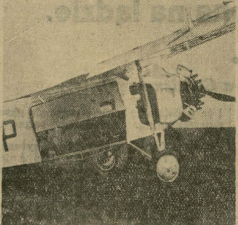
Samolot sanitarny Lublin R. XVI. Otwarcie kabiny dla załadunku chorych na noszach. Z przodu widoczne osobne wejście dla pilota i mechanika
