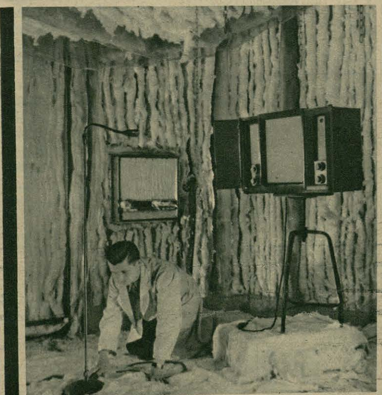
PROBA CZYSTOŚCI DŹWIEKÓW W APARACIE RADJOWYM. Ażeby z jak najdalej idącą dokładnością wypróbować czystość dźwiękową aparatów radiowych, wyścieliła się w laboratorium ścianą grubą warstwą waty, która nie dopuszcza żadnych szmerów z zewnątrz. Wszystkie potrzebne do badania przyrządy umieszczone są poza takimi ścianami z waty.
