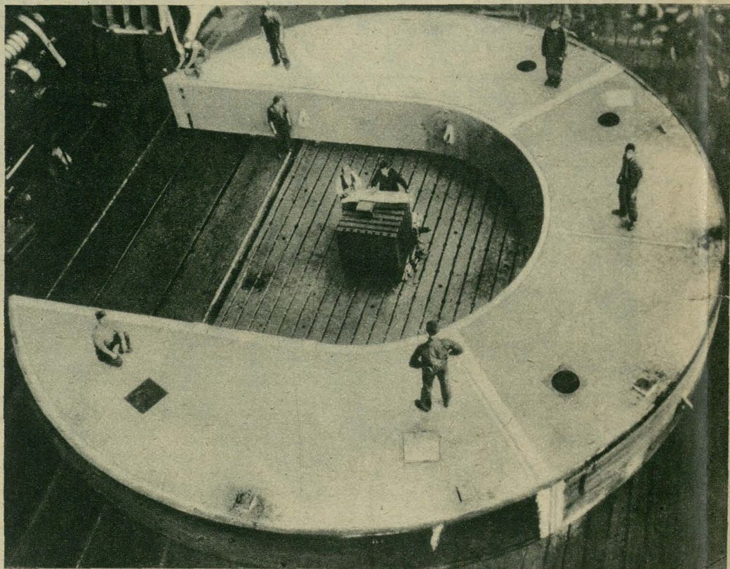
BUDOWA OLBRZYMIEGO TELESKOPU. W warsztatach w Pittsburgu przeprowadza się obecnie konstrukcję olbrzymiego teleskopu, przeznaczonego dla obserwatorium na Mount Palomar w Kalifornji. W tym celu zbudowano łożysko o niebywałych rozmiarach — 14 m średnicy i olbrzymim ciężarze — 317.000 funt.
