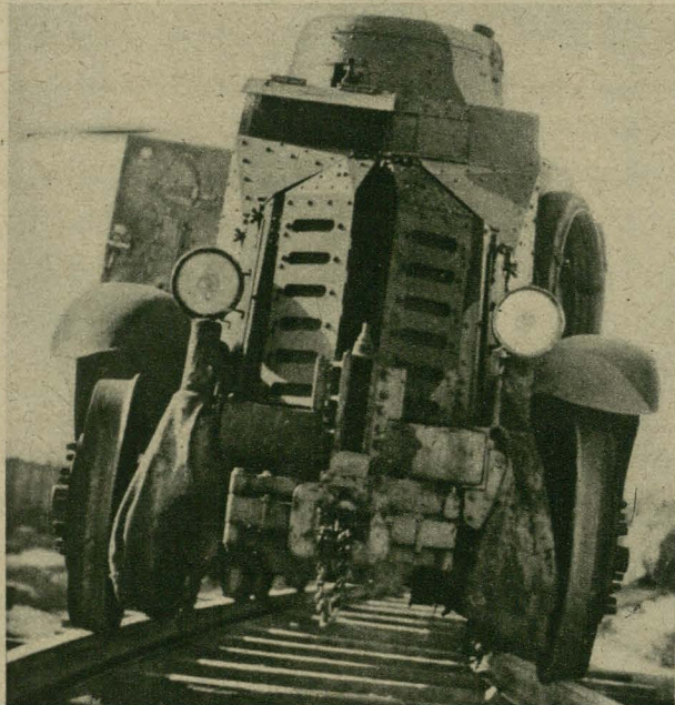
JAPONCZYCY NA FRONCIE CHIŃSKIM posługują się najnowszym ryszunkiem wojennym, odnosząc duże sukcesy m. in. również dzięki transportowi wojsk w potężnych pociągach pancernych.
