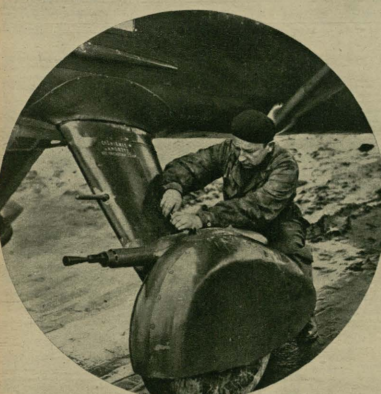
Karabin maszynowy wmontowany w goleń podwozia samolotu pościgowo-bombowego.
