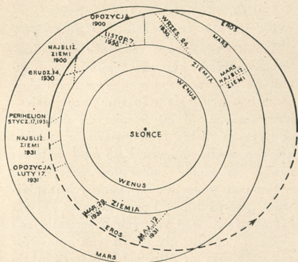
Orbity: Wenus, Ziemi, Erosa i Marsa. Linie proste łączą współczesne położenia Ziemi i Erosa.
