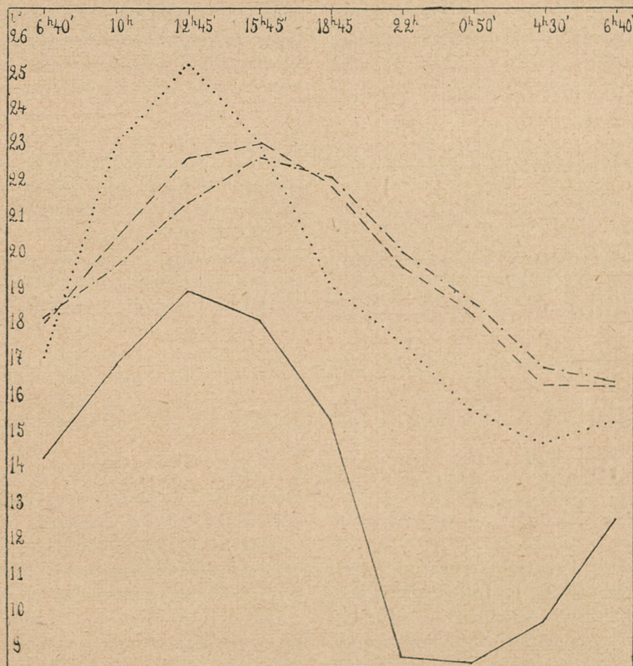
Rys. 2. Przebieg temperatury wody w zbiorniku niezacienionym w czasie doby (30.VI—1.VII). Linia ciągła — temp. powietrza, przerywana — temp. powierzchni wody, kreski i kropki — temp. wody na głębokości 30 cm., kropkowana — temp. wody przybrzeżnej.
