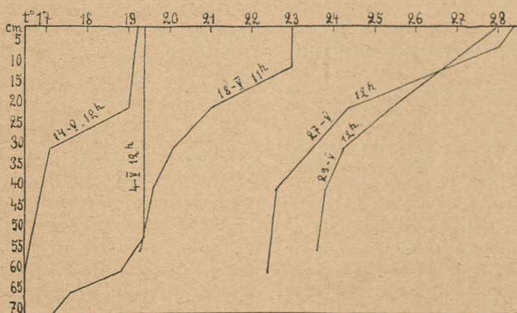
Rys. 3. Występowanie skoku termicznego w płytkim zbiorniku wodnym.
