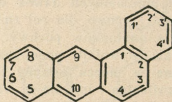
1,2-BENZANTRACEN
