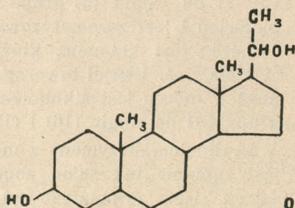
PREGNANDIOL
