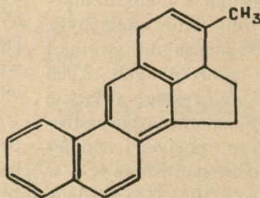
METYLOCHOLANTREN
