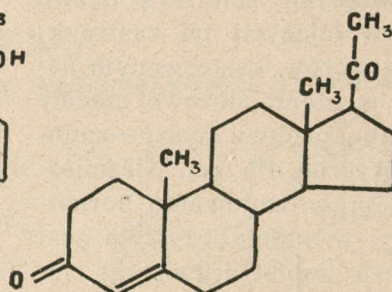
PROGESTERON
