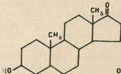
ANDROSTERON
