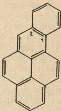
1,2-BENZPYREN
