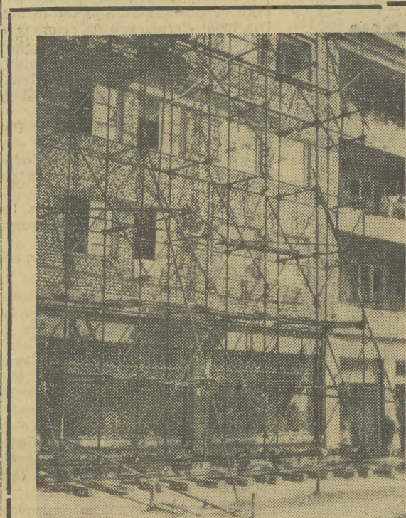
Przy budowie Osiedla A-Zachód zastosowano nowy system przy tynkowaniu zewnętrznych murów. System polega na przesuwaniu wzdłuż murów części rusztowania skonstruowanego z stalowych rur. System ten jest bardzo praktyczny i przynosi duże oszczędności.
