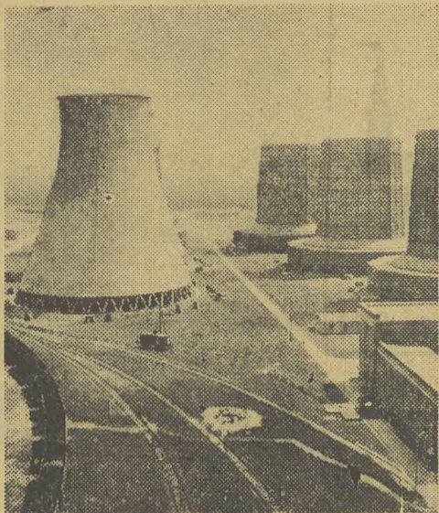
W Skawinie przystąpiono do drugiego etapu budowy silowni. Po uruchomieniu generatorów mniejszych, przystąpiono obecnie do montażu największego w Polsce generatora. Ukończenie prac montażowych przewidziane jest w końcu br. CAF — Tyminski
