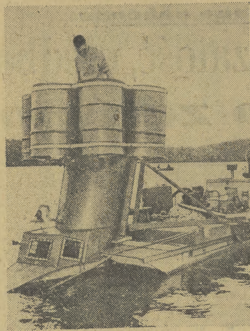
Wydział Biologii Uniwersytetu w Wisconsin (USA) dysponuje takim oto pływającym sprzętem, umożliwiającym obserwację podwodnego życia. Zanurzenie kabiny uzależnione jest od stopnia wypełnienia górnych zbiorników wodą. (db)
