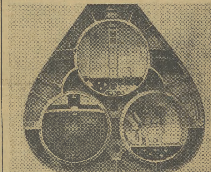
Co to? Przekrój bardzo pomysłowego wnętrza podwodnej łodzi. Projekty pierwszych takich modeli pokazano ostatnio na wystawie w Amsterdamie.
