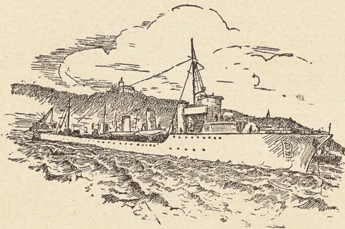
To torpedowce...
